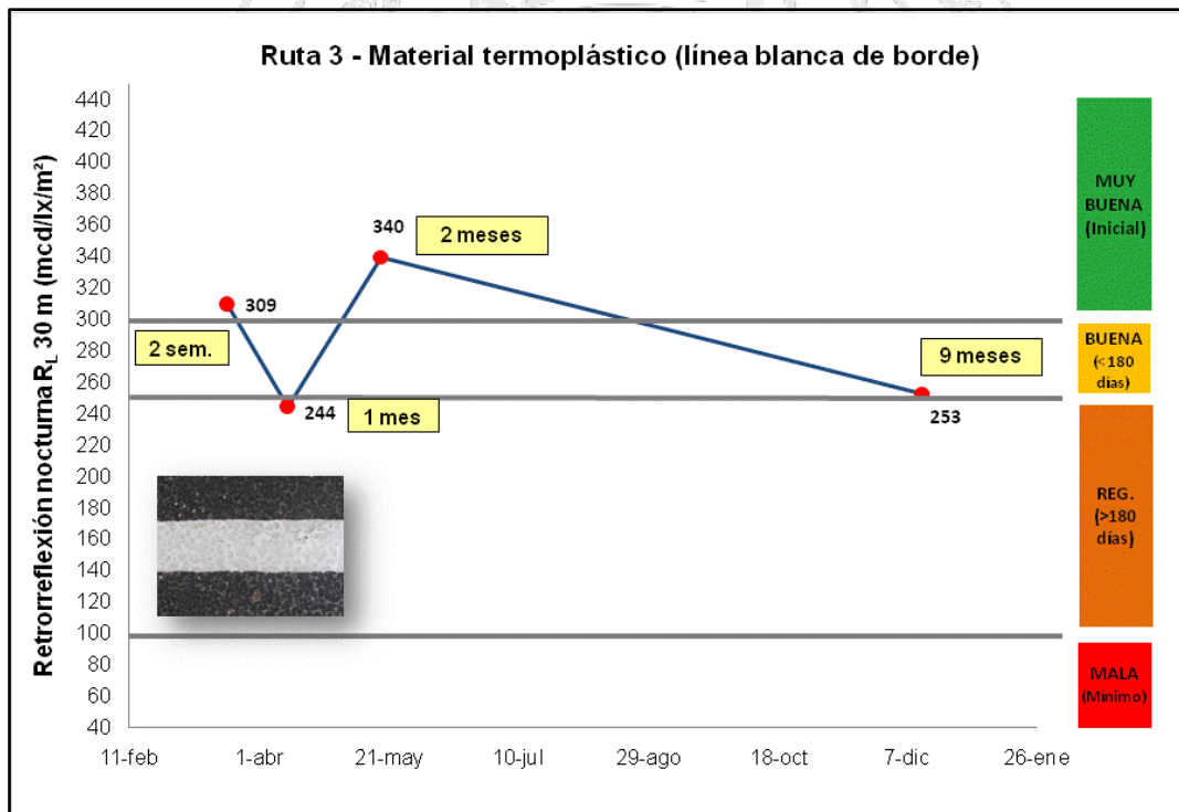
Figura 9.9. Retrorreflexión con equipo manual de línea blanca de borde, Ruta 3.
