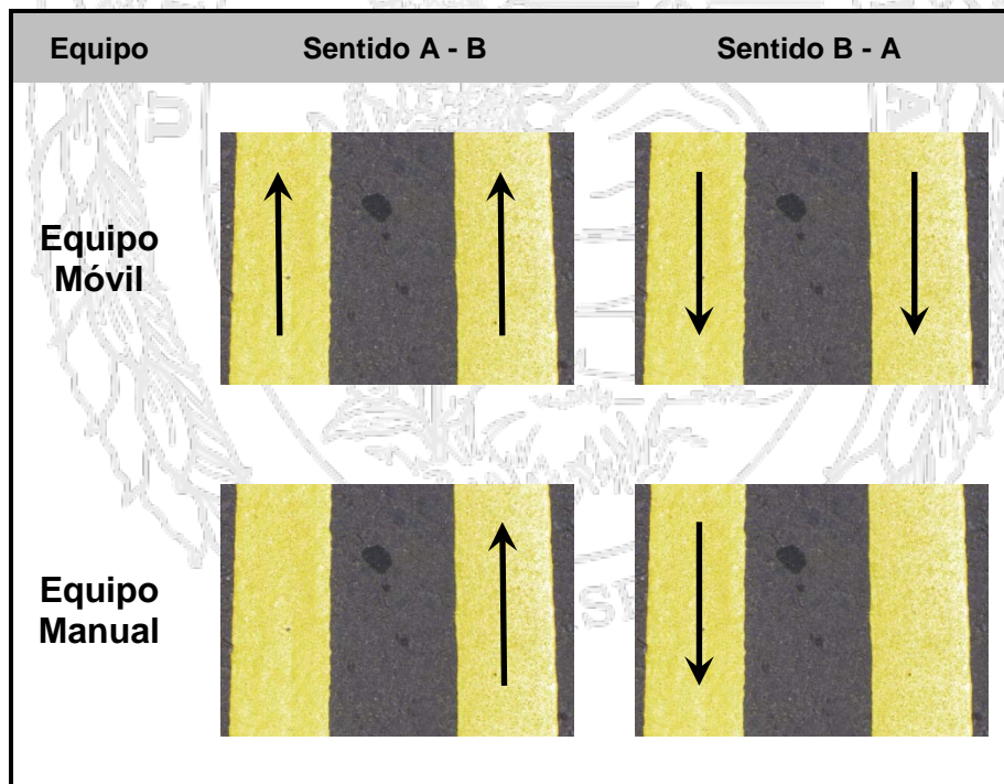
Figura 8.6. Esquema de medición de doble línea amarilla con equipo manual y móvil.
