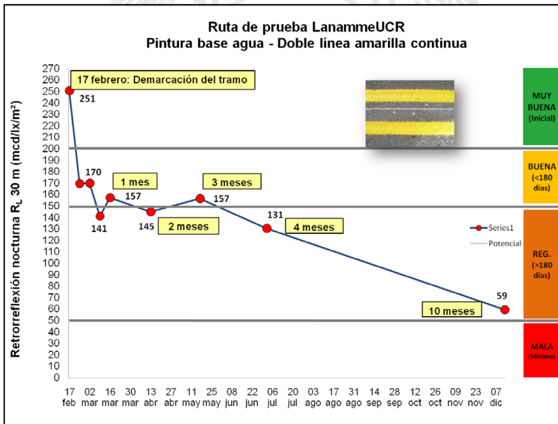
Figura 9.8. Gráfico de retrorreflexión horizontal, ruta de travesía LanammeUCR.
