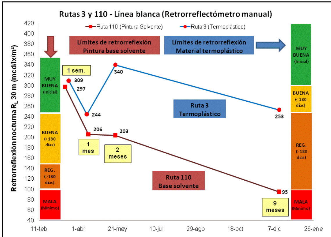
Figura 9.17. Comparación de retroreflexión de termoplástico y base solvente, línea blanca.
