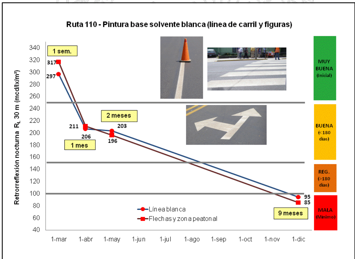
Figura 9.14. Retrorreflexión con equipo manual de líneas blancas y figuras, Ruta 110.
