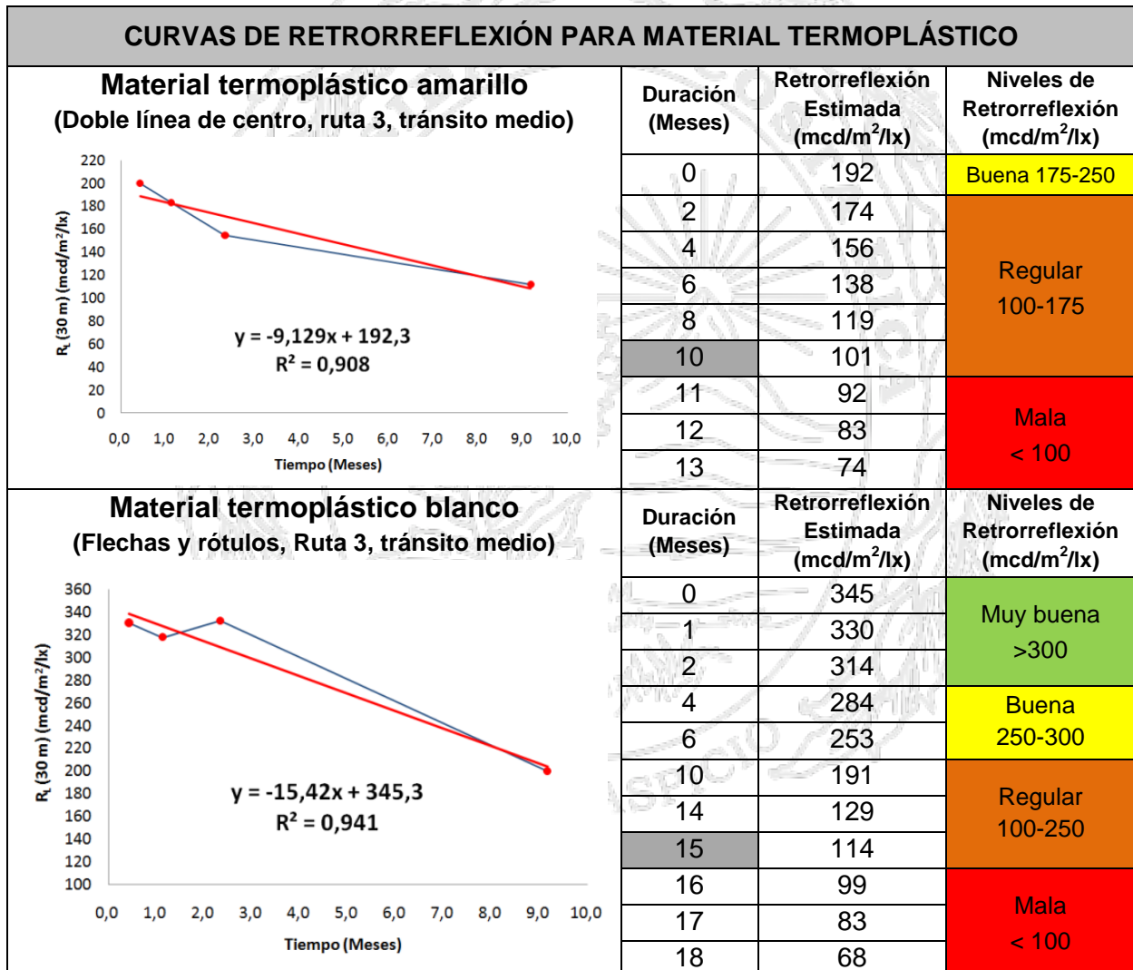
Figura 9.19. Curvas de mejor ajuste para material termoplástico.
