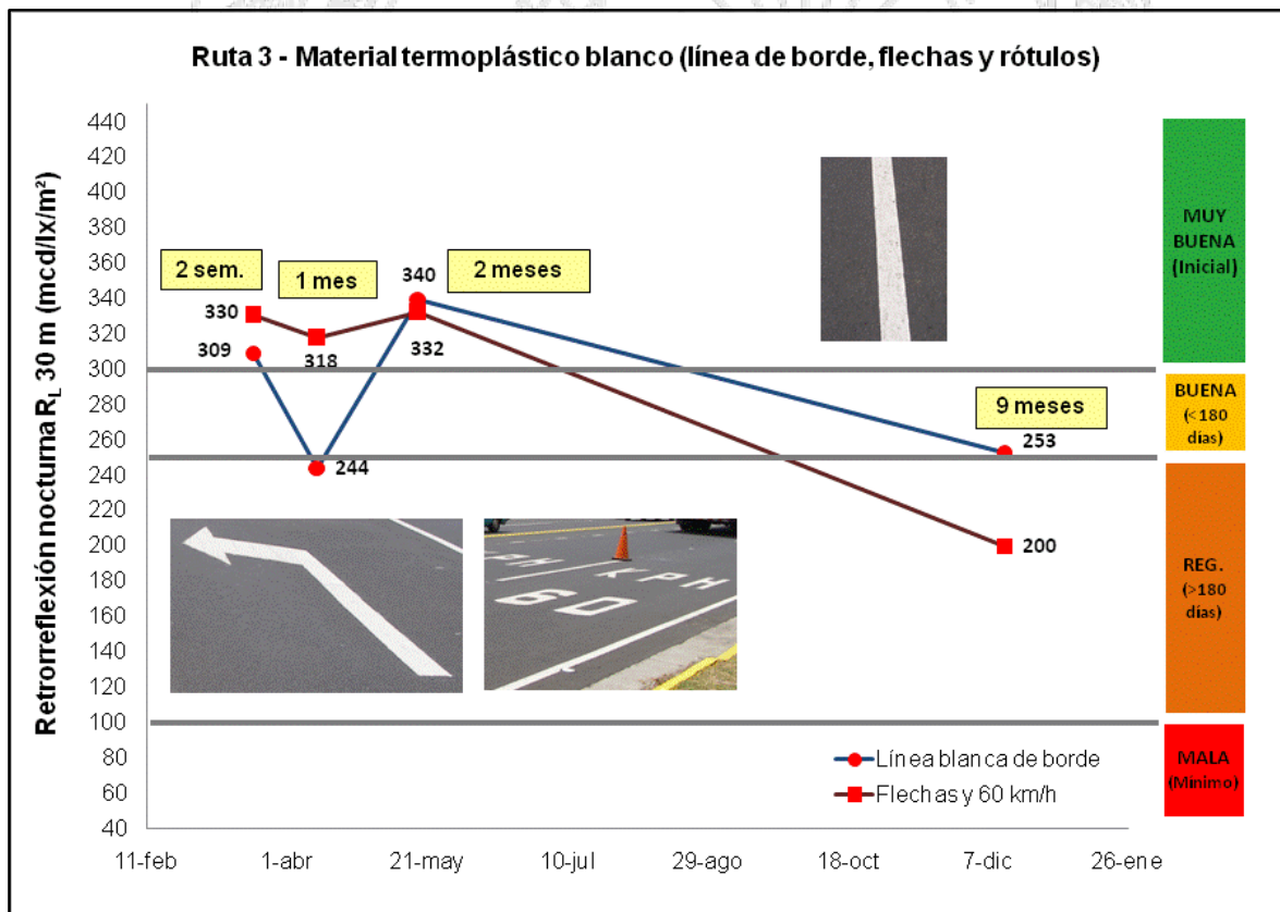
Figura 9.11. Retroreflexión con equipo manual de líneas blancas, figuras y rótulos, Ruta 3.
