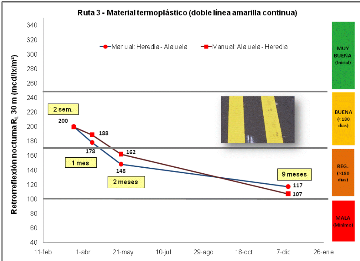
Figura 9.10. Retroreflexión con equipo manual de línea amarilla de centro, Ruta 3.
