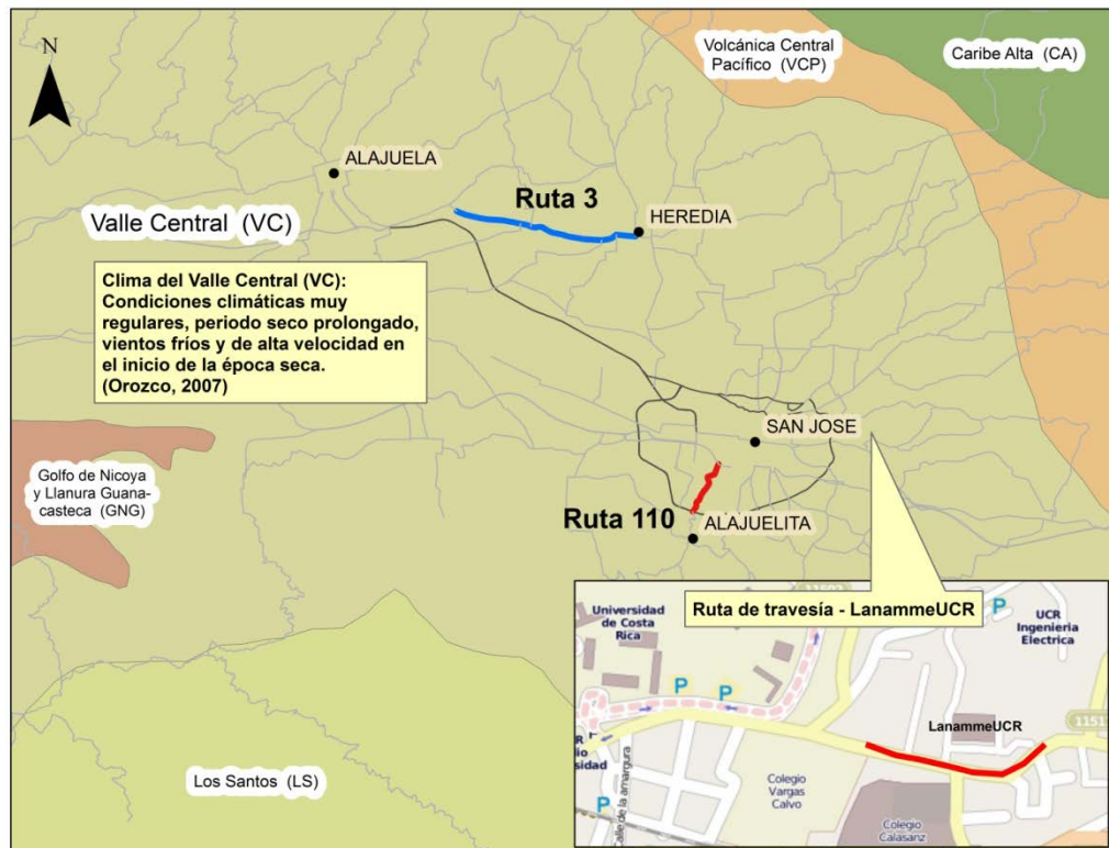
Figura 8.1. Secciones de estudio de las rutas nacionales 3, 110 y la ruta de travesía LanammeUCR para mediciones del parámetro de retroreflexión.
