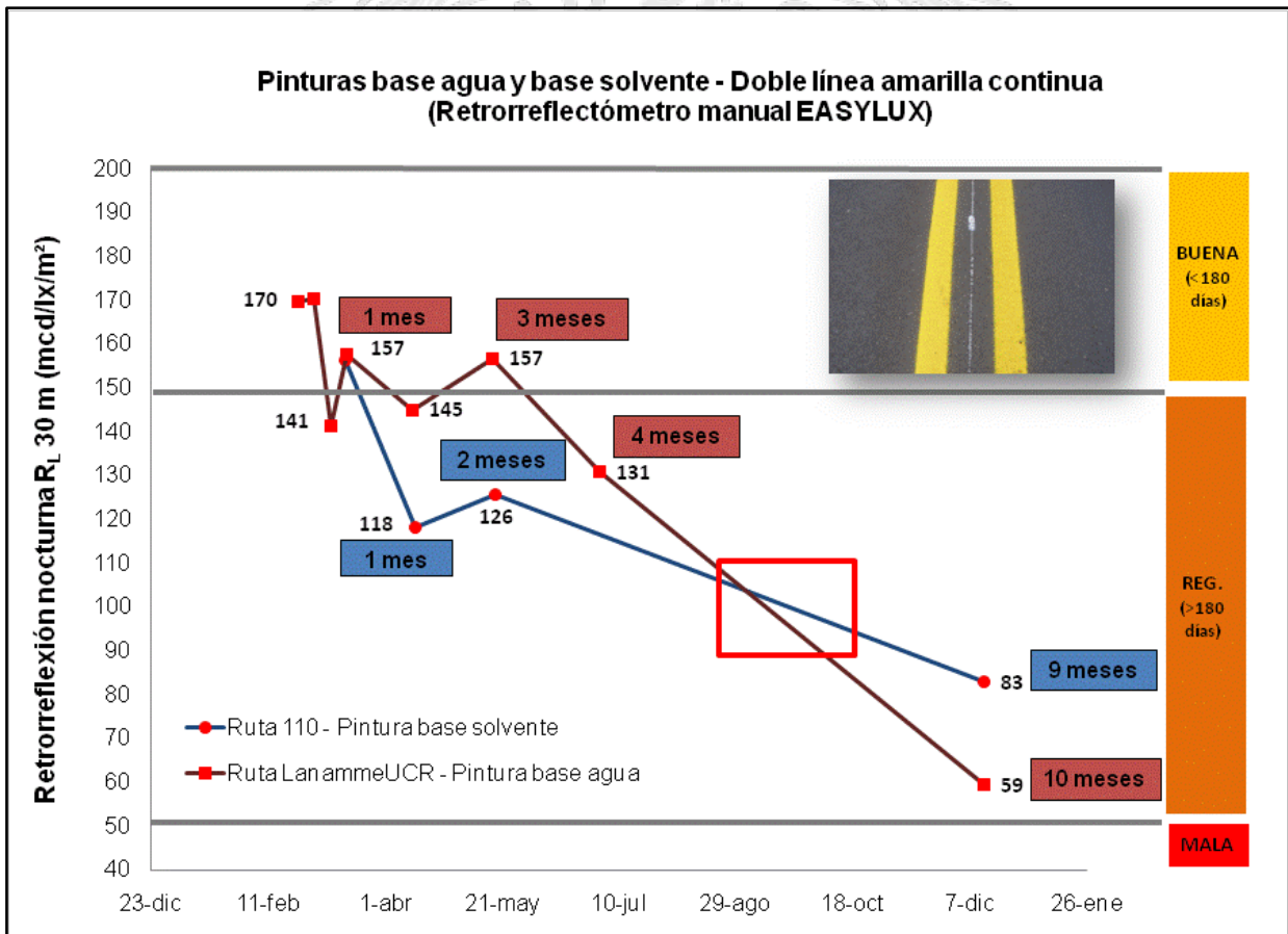
Figura 9.15. Comparación de retroreflexión de pinturas base agua y base solvente.
