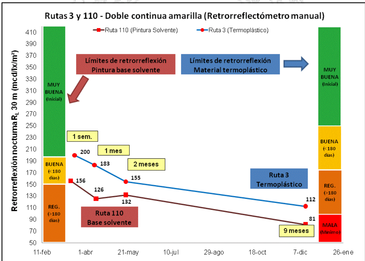
Figura 9.16. Comparación de retroreflexión de termoplástico y base solvente, línea amarilla.
