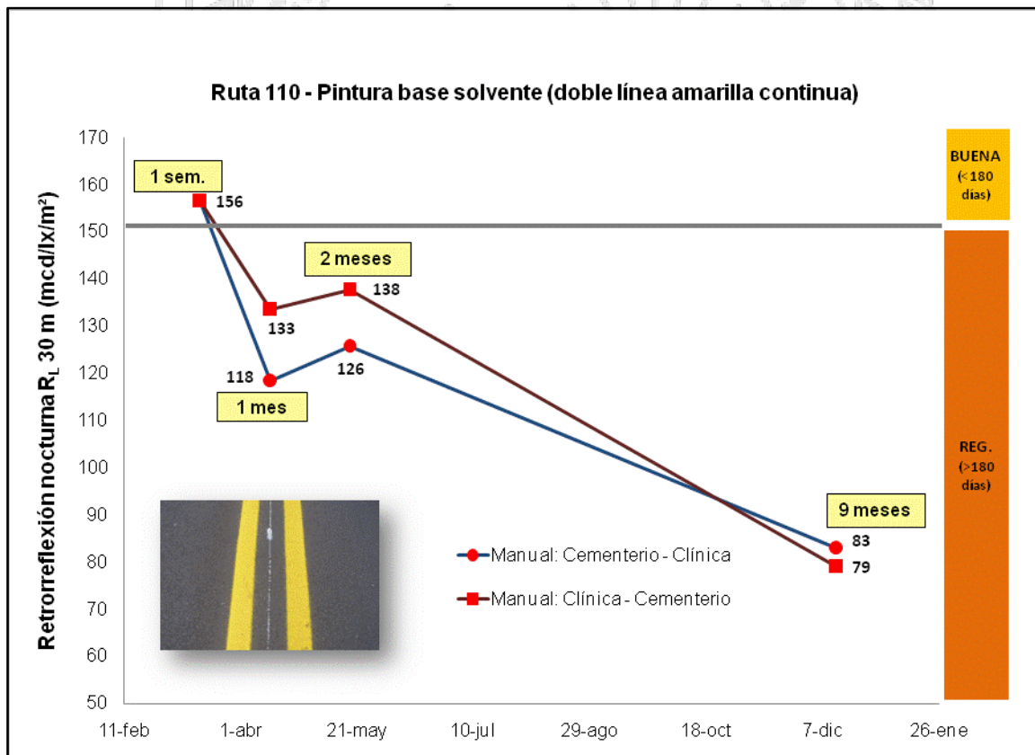
Figura 9.13. Retrorreflexión con equipo manual de línea central amarilla, Ruta 110.
