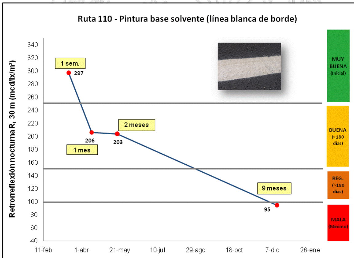
Figura 9.12. Retrorreflexión con equipo manual de línea blanca de borde, Ruta 110.
