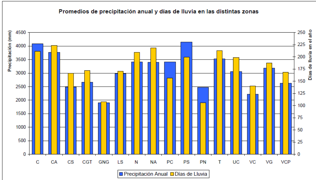
Figura 7.6. Gráfico de promedios de precipitación anual y días de lluvia en Costa Rica.
