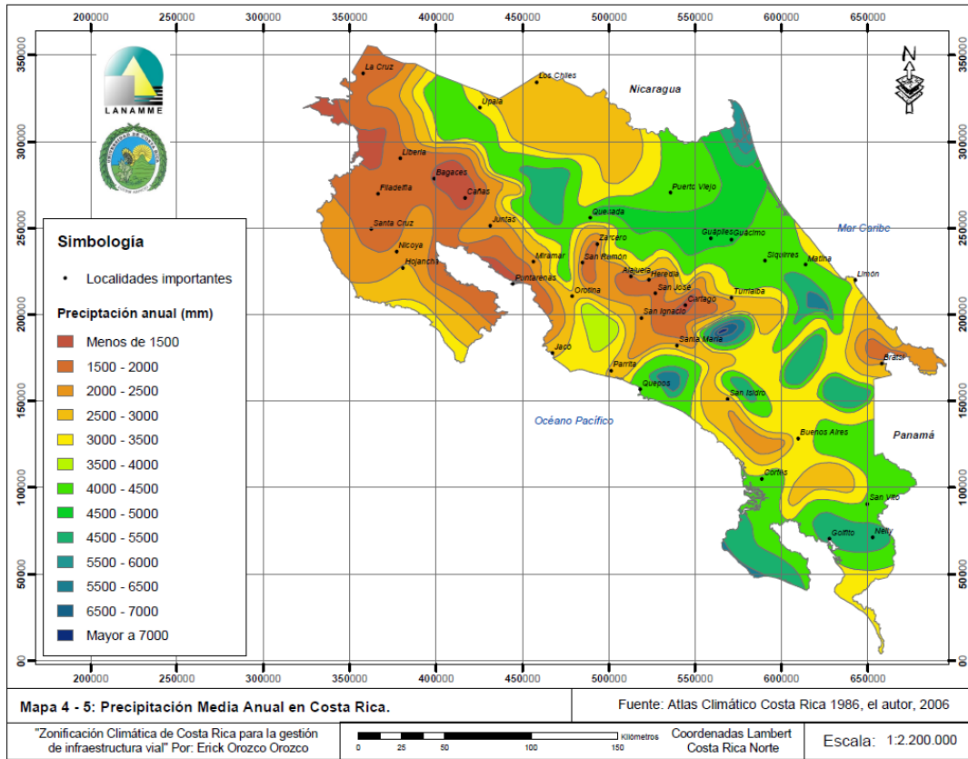
Figura 7.3. Mapa de precipitación media anual en Costa Rica.
