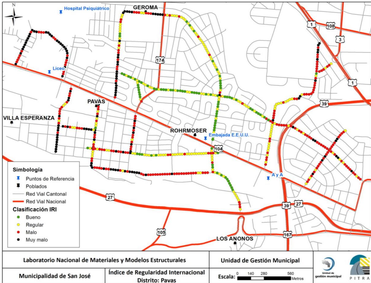
Figura 10. Condición del IRI para las mediciones realizadas en Pavas.
