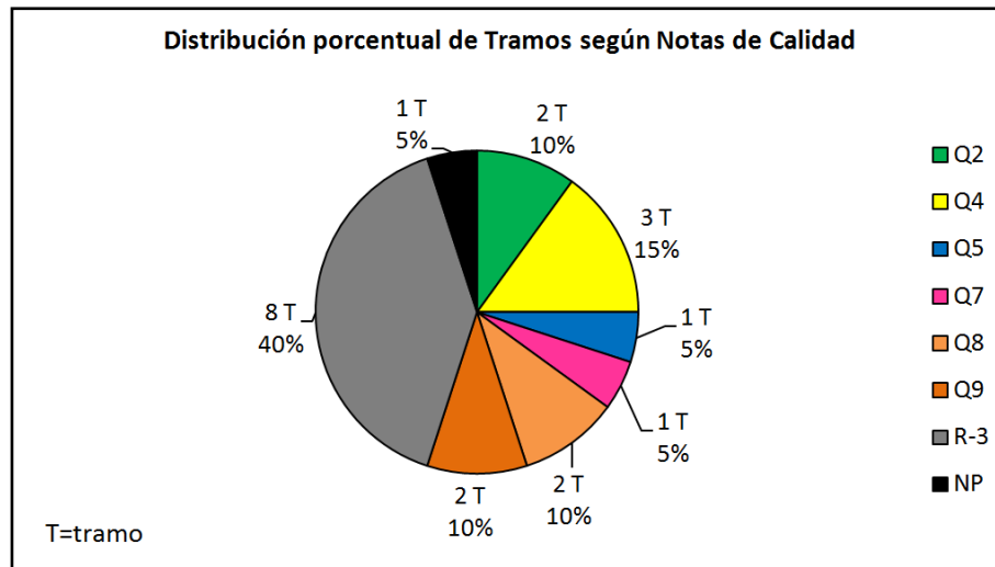
Figura 25. Distribución porcentual de las notas de calidad asignadas a cada sección analizada.
