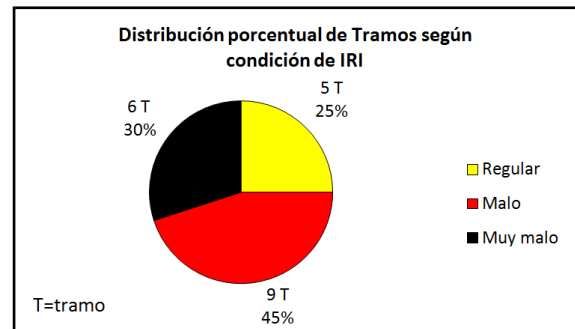
Figura 23. Porcentaje de tramos clasificados según el IRI promedio.
