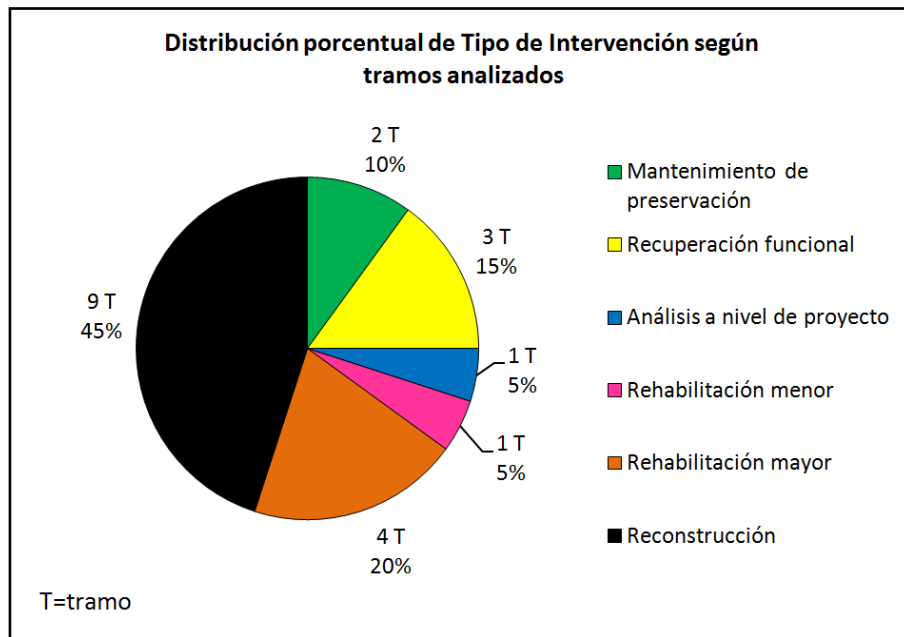
Figura 28. Tipos de intervención requerida para la red vial cantonal de Pavas, según cantidad de tramos.
