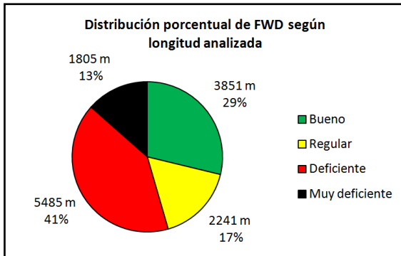
Figura 19. Porcentaje de metros lineales clasificados según FWD promedio.
