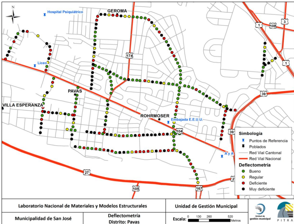
Figura 15. Condición del FWD para las mediciones realizadas en Pavas.
