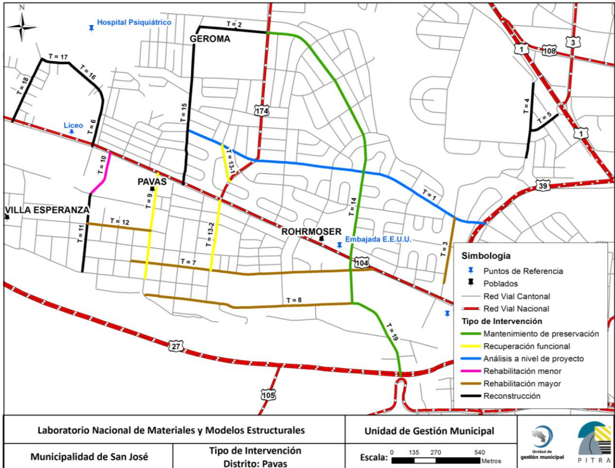
Figura 29. Tipo de intervención recomendado para cada tramo analizado.
