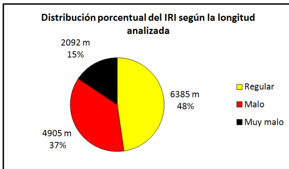
Figura 22. Porcentaje de metros lineales clasificados según el IRI promedio.
