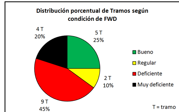
Figura 20. Porcentaje de tramos clasificados según el FWD promedio.
