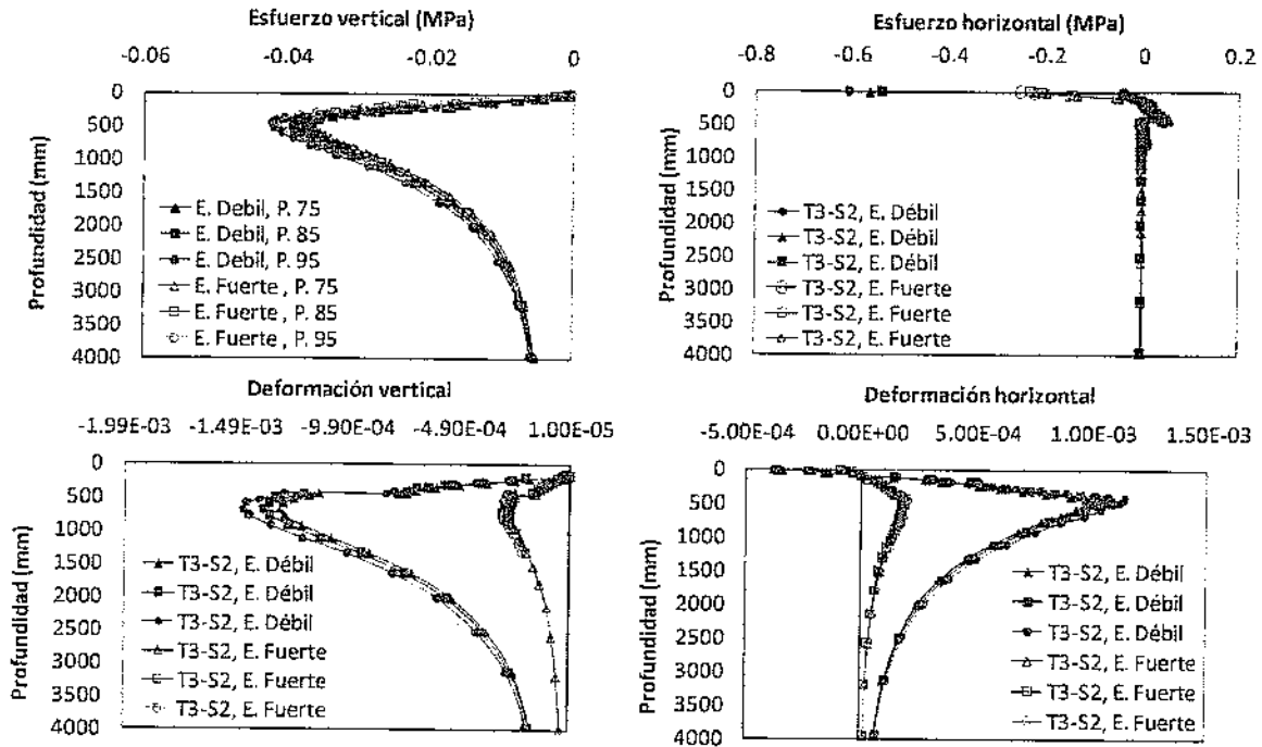
Figura 4: Esfuerzos y deformaciones configuración T3-S2 tándem
