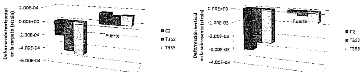
Figura 7: Deformación horizontal y vertical en los puntos críticos de la sección estructural para el Percentil 95 de carga
