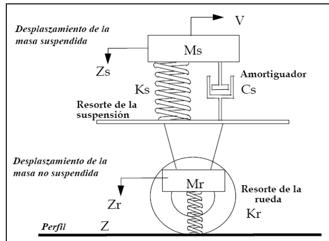
Figura 1.- Modelo de cuarto de carro. Fuente: (De Solminihaç, 2006)
