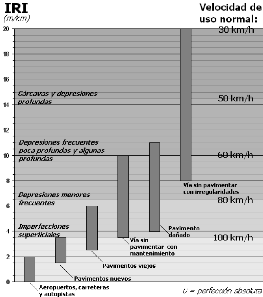
Figura 2.- Escala estándar empleada por el Banco Mundial para la cuantificación del IRI para diferentes tipos de vías. Fuente: (Adaptado de UMTRI Research Review, 2002)
