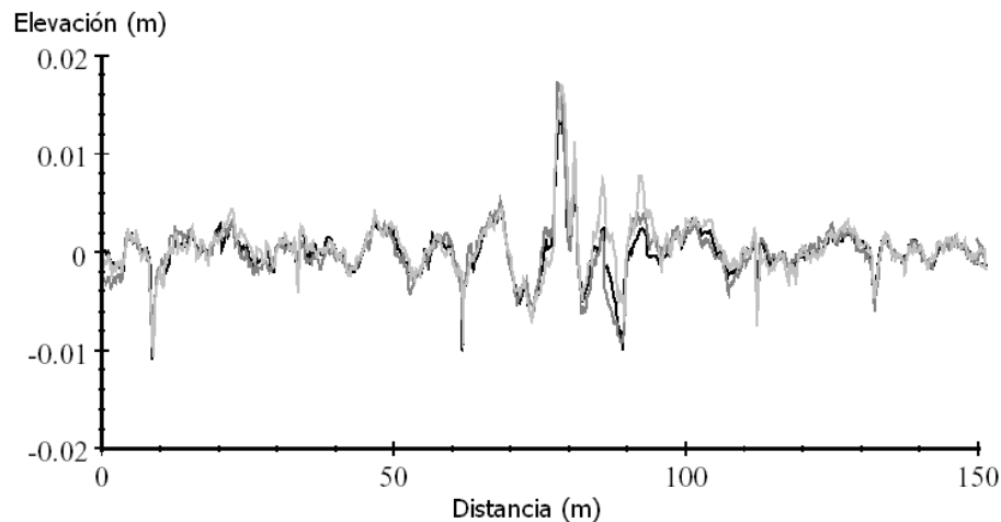
Figura 4.- Los mismos perfiles de la figura anterior después del filtrado. Fuente: (Sayers & Karamihas, 1998)
