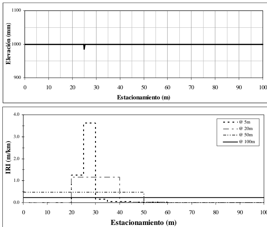
Figura 6.- Simulación de una junta de construcción. Fuente: (El Autor)
