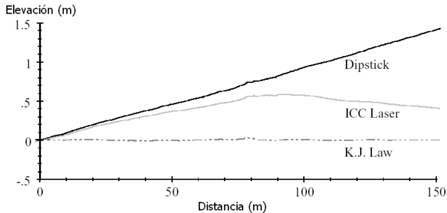
Figura 3.- Variaciones aparentes de perfiles longitudinales utilizando diferentes equipos. Fuente: (Sayers & Karamihas, 1998)
