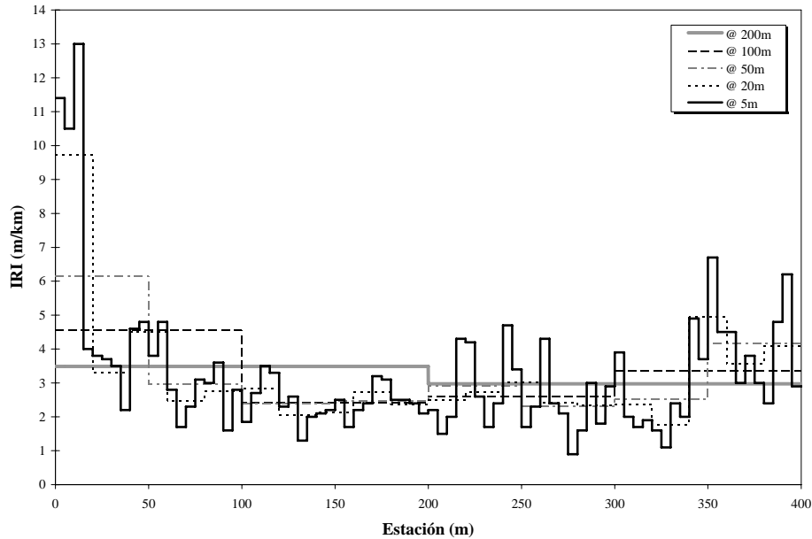
Figura 5.- Variación en el valor del IRI según la longitud de evaluación. Fuente: (El Autor)
