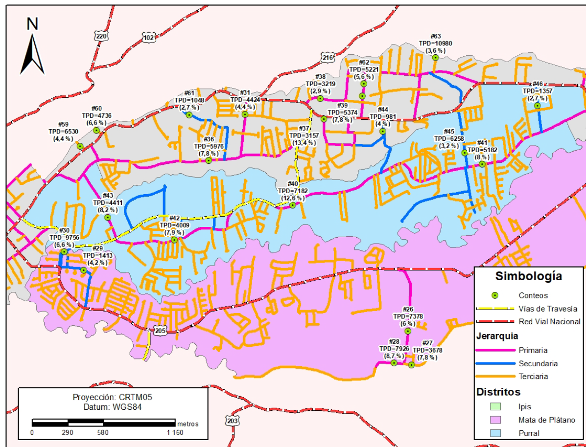
Figura 3. Conteo vehiculares realizados en los distritos de Ipís, Purral y Mata de Plátano.
