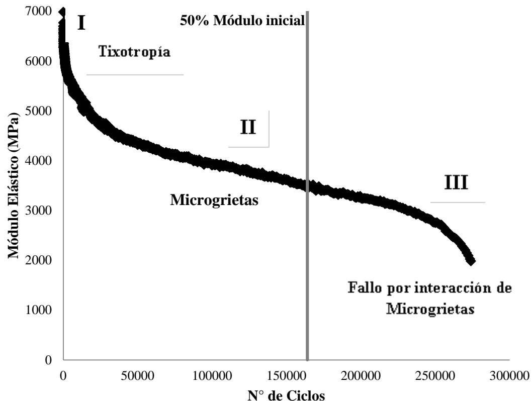
Figura 16. Curva de fatiga a deformación controlada de mezcla asfáltica medida en el laboratorio, preparada con asfalto Costa Rica 2
