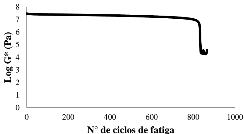
Figura 19. Ensayo de Fatiga a Esfuerzo Controlado
