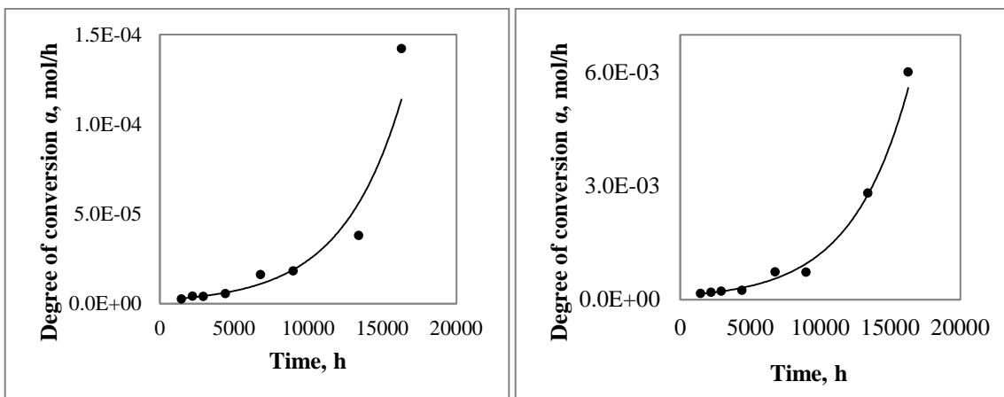
Figura 10. Comportamiento cinético de la producción de a) carbonilos y b) sulfóxidos mediante el mecanismo D1 para el betún expuesto a condiciones ambientales
