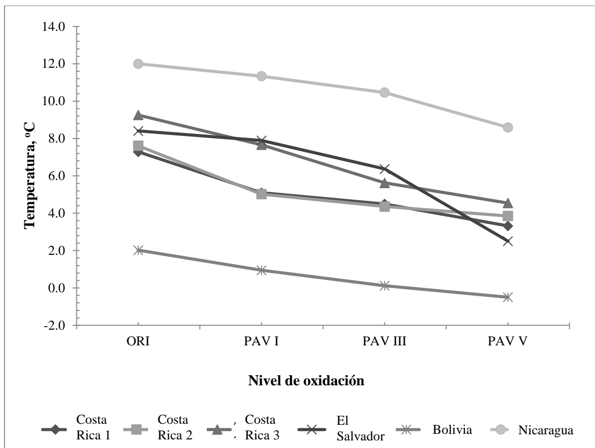
Figura 3. Temperaturas de transición vítrea para seis betunes diferentes y cuatro grados de oxidación (desde original hasta 5 ciclos PAV)
