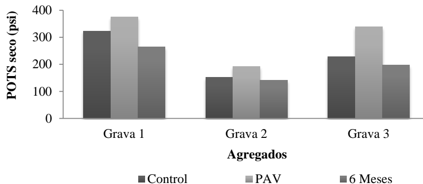
Figura 26. Valores de POTS para las combinaciones betún-agregado
