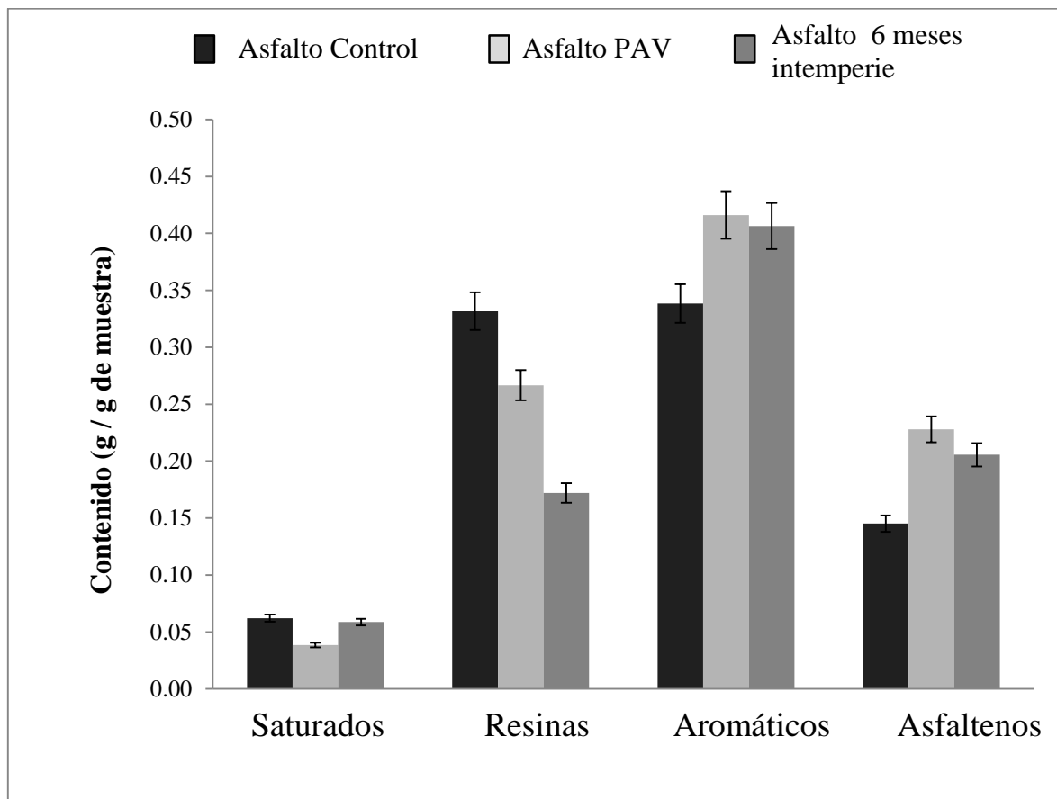
Figura 6. Contenido de las fracciones SARA en las muestras de betún control y oxidados.
