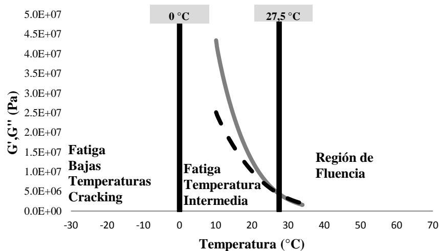
Figura 14. Variación del componente elástico, G' (línea gris) y componente viscoso G'' (línea negra) con temperatura en a) aglutinante no oxidado, b) aglutinante envejecido en RTFO y c) Betún oxidado PAV.
