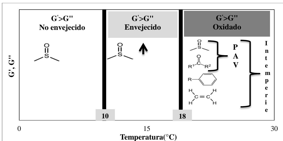
Figura 24. Método RHEO-PLUS, evaluación reológica del nivel de envejecimiento y oxidación del betún y su relación con la composición química.
