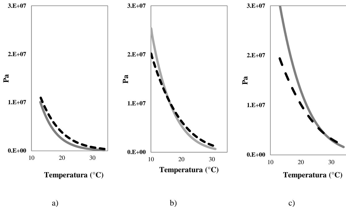
Figura 13. Variación del componente elástico, G' (línea gris) y componente viscoso G'' (línea negra) con temperatura en a) aglutinante no oxidado, b) aglutinante envejecido en RTFO y c) Betún oxidado PAV.
