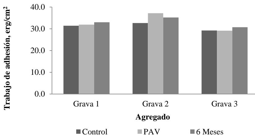
Figura 25. Trabajo de adhesión entre los betunes control y oxidados y distintas gravas
