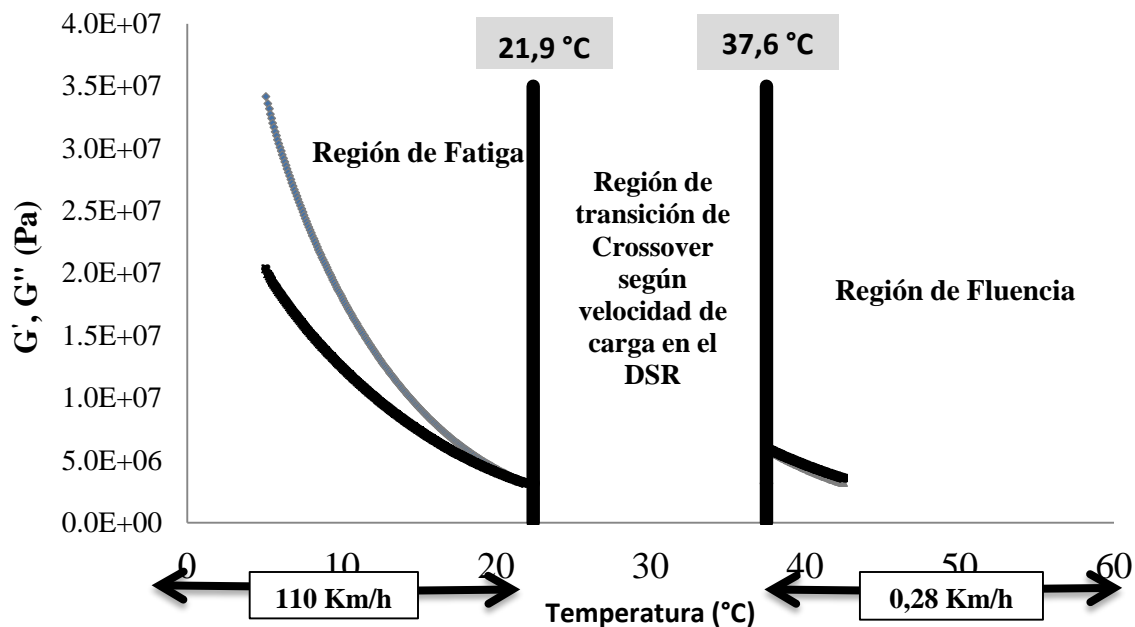
Figura 15. Influencia de la velocidad de carga sobre la temperatura de Crossover para el betún Costa Rica 2 PAV
