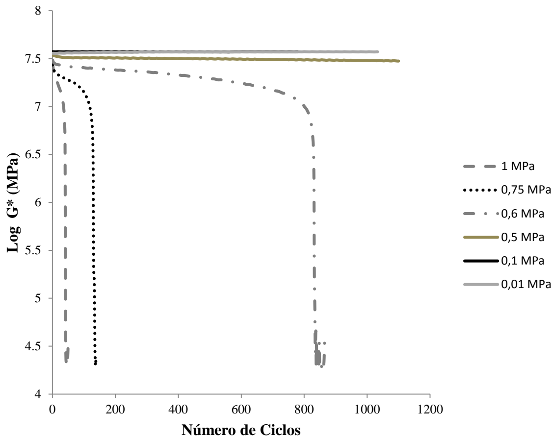
Figura 22. Barrido de esfuerzos para determinación de la carga en el ensayo de Fatiga a Esfuerzo Controlado
