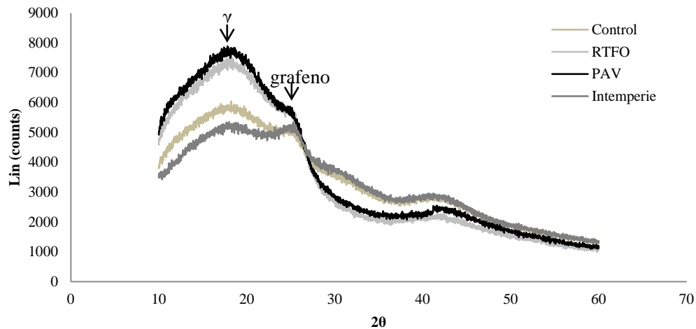
Figura 7. Diffractogramas de los asfaltenos control y oxidados
