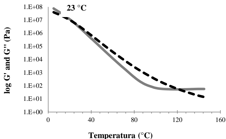
Figura 12. Variación de la componente elástica G' (línea gris continua) y la componente viscosa G'' (línea negra de puntos) con temperatura para una muestra de betún oxidado en campo durante seis meses
