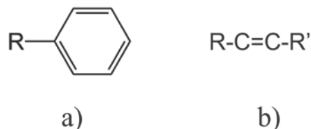
Figura 5. (a) Aromáticos y (b) enlaces dobles carbono-carbono
