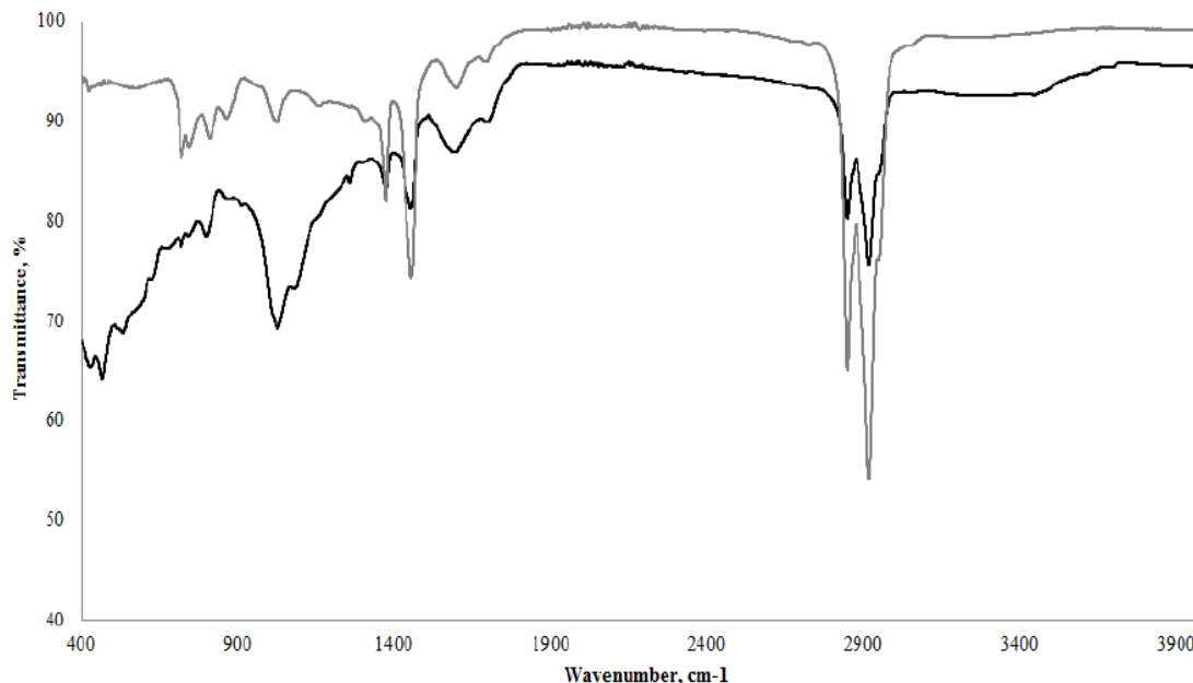
Figura 9. Espectro de infrarrojo del betún luego de oxidación en el laboratorio (línea gris) y en el campo (línea negra)
