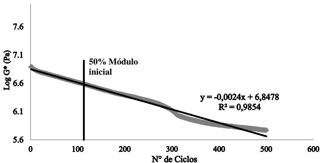
Figura 17. Ensayo clásico de fatiga a deformación controlada para el betún Costa Rica 2 en el DSR
