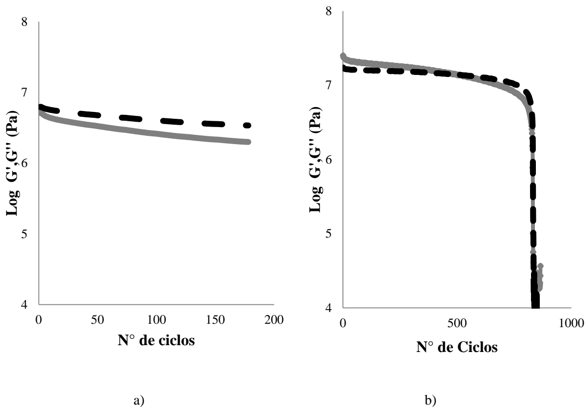
Figura 21. Comparación del comportamiento de las componentes elástica, G' (gris) y viscosa, G'' (negra) en el ensayo de Fatiga a) a deformación controlada (10%) y b) a esfuerzo controlado (0,6 MPa) del betún Costa Rica 2
