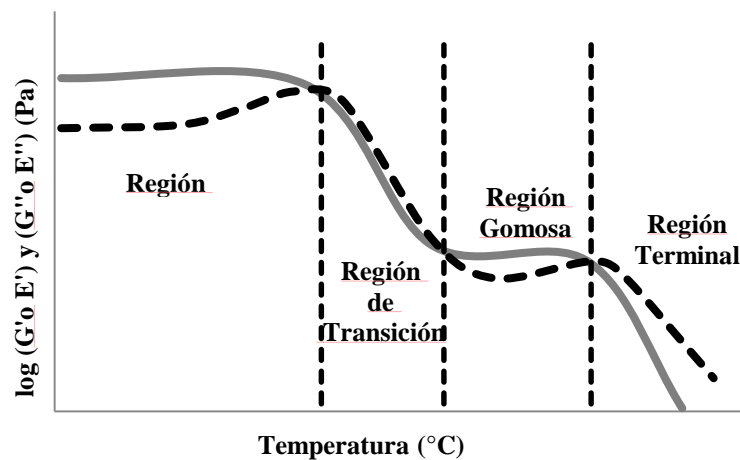
Figura 11. Regiones del comportamiento viscoelástico de un polímero, donde se observa la variación de la componente elástica G' (línea gris continua) y la componente viscosa G'' (línea negra de puntos) con temperatura
