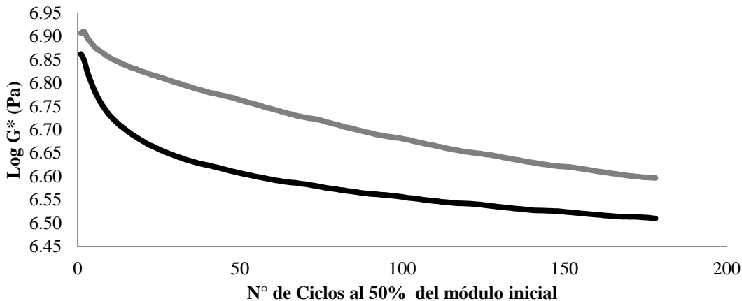
Figura 18. Recuperación de módulo luego de una hora de reposo (línea negra) tras el ensayo de fatiga convencional (línea gris).
