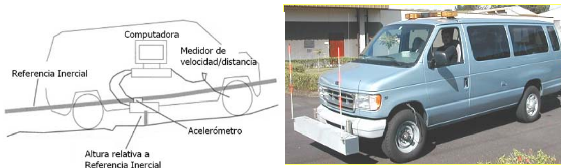
Figura 13. Perfilómetro Inercial Láser (Fuente: LanammeUCR, 2008).
