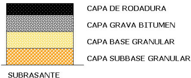
Figura 18. Ejemplo de estructura de pavimento.
