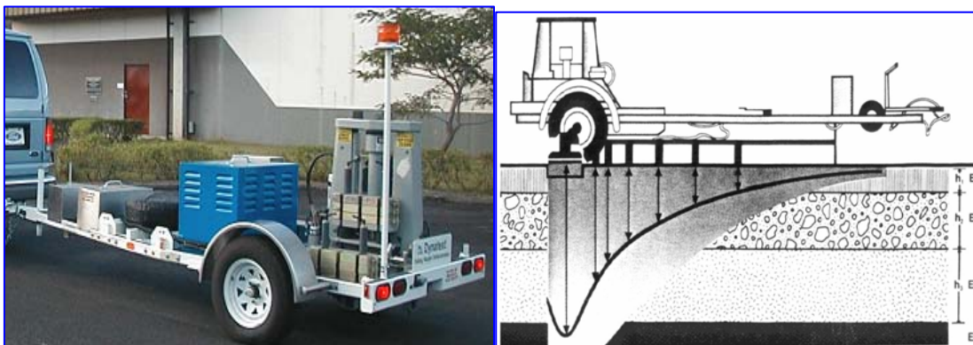
Figura 15. Equipo de deflectometría de impacto (Fuente: LanammeUCR, 2008).
