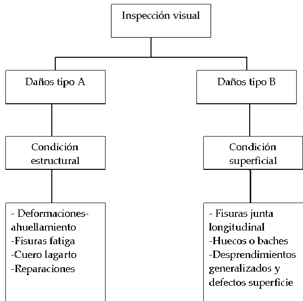
Figura 5. Esquema de inspección visual en metodología VIZIR (Fuente: LanammeUCR, 2008).
