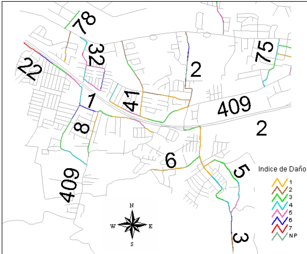
Figura 11. Índice de Daño de la RVC de La Unión, sector Sur Oeste (Fuente: LanammeUCR, 2009).
