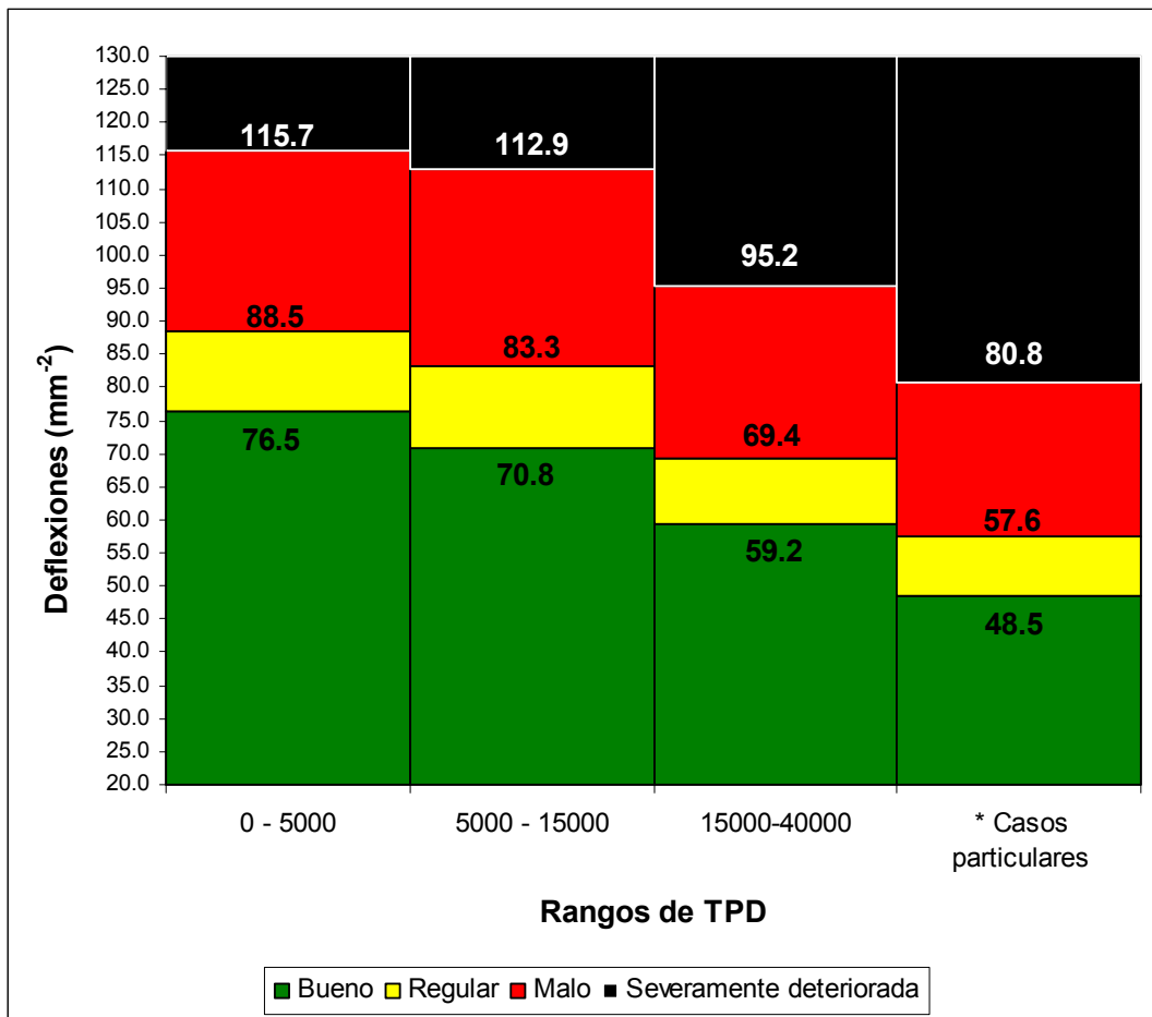
Figura 16. Condición del pavimento a partir de deflectometría y TPD, para una base granular. (Fuente: LanammeUCR, 2008).
