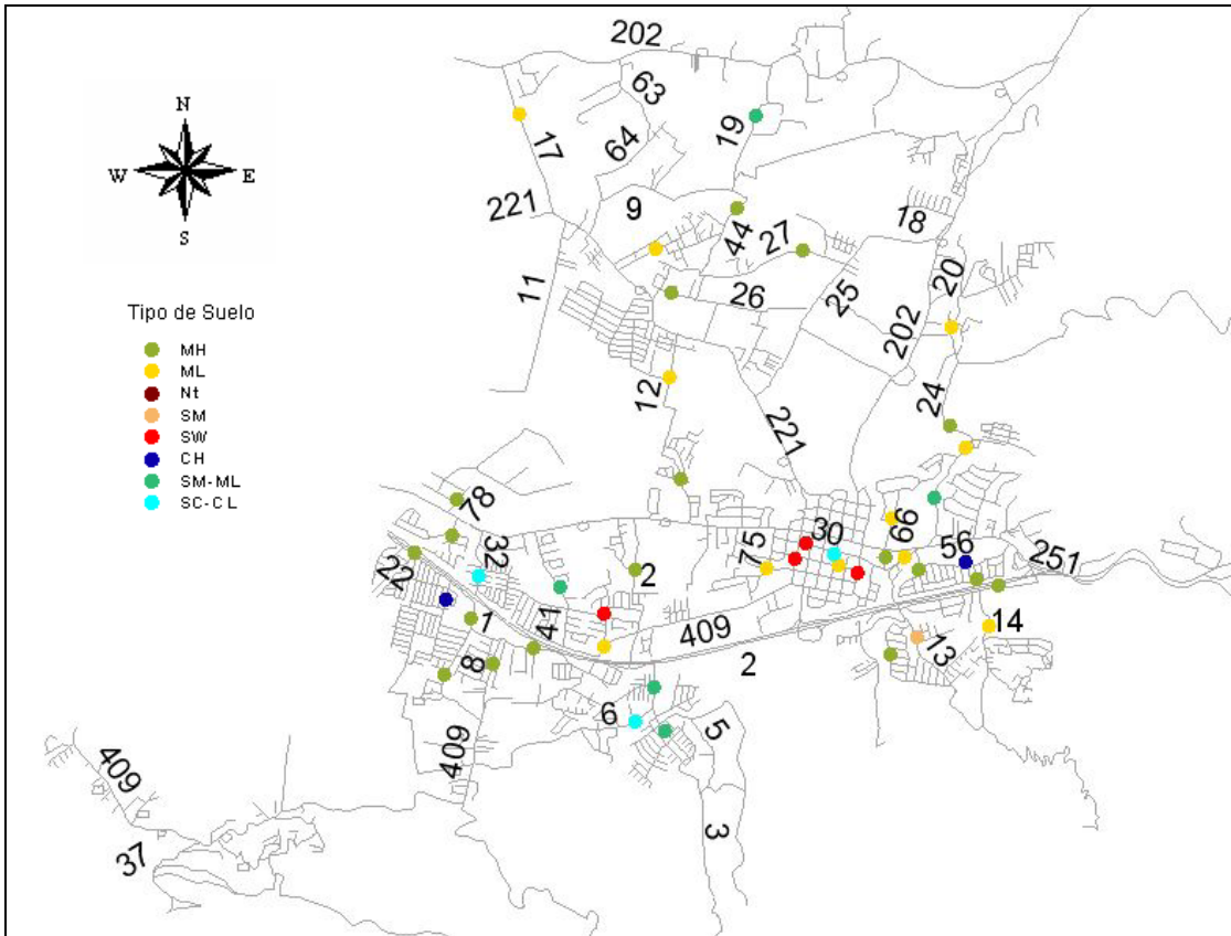
Figura 20. Tipo de suelo para la sub-rasante en el cantón de La Unión (Fuente: LanammeUCR, 2009).
