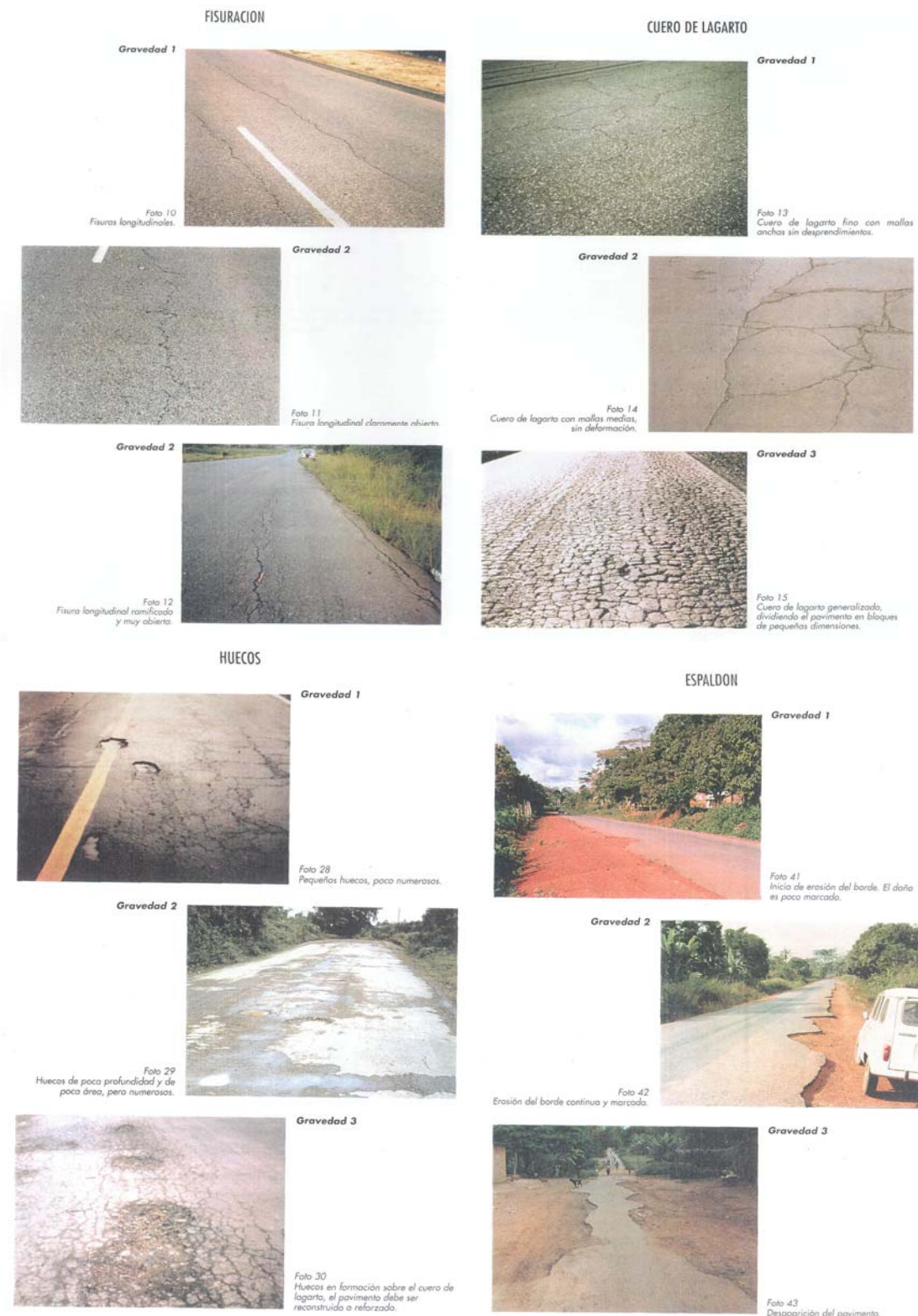
Figura 7. Ejemplos de daños superficiales con metodología VIZIR (Fuente: VIZIR, técnicas y métodos).
