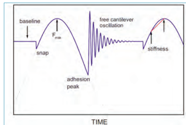
Figura 3. Operación PFM. Fuente: Witec, modificado por autores.
