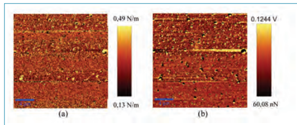
Figura 7 Mediciones PFM de resinas en asfalto PG64-22: a) rigidez y b) adhesión.
