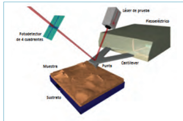
Figura 2. Funcionamiento del AFM. Fuente: Witec, modificado por autores.
