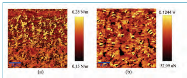
Figura 8 Mediciones PFM de aromáticos en asfalto PG64-22: a) rigidez y b) adhesión.
