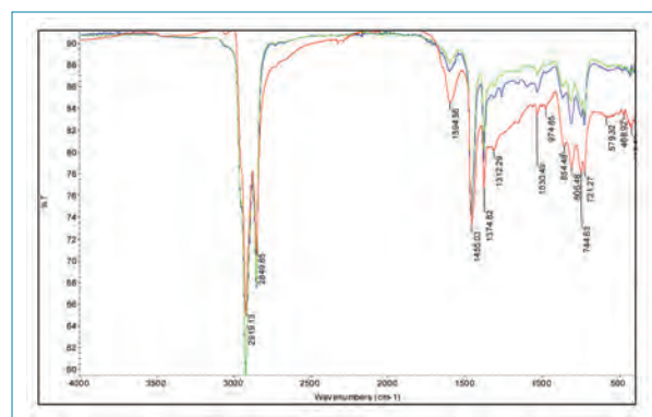
Figura 9 Análisis FTIR del asfalto y sus componentes (Azul=asfalto PG64-22, Rojo=asfaltenos, Verde=maltenos).
