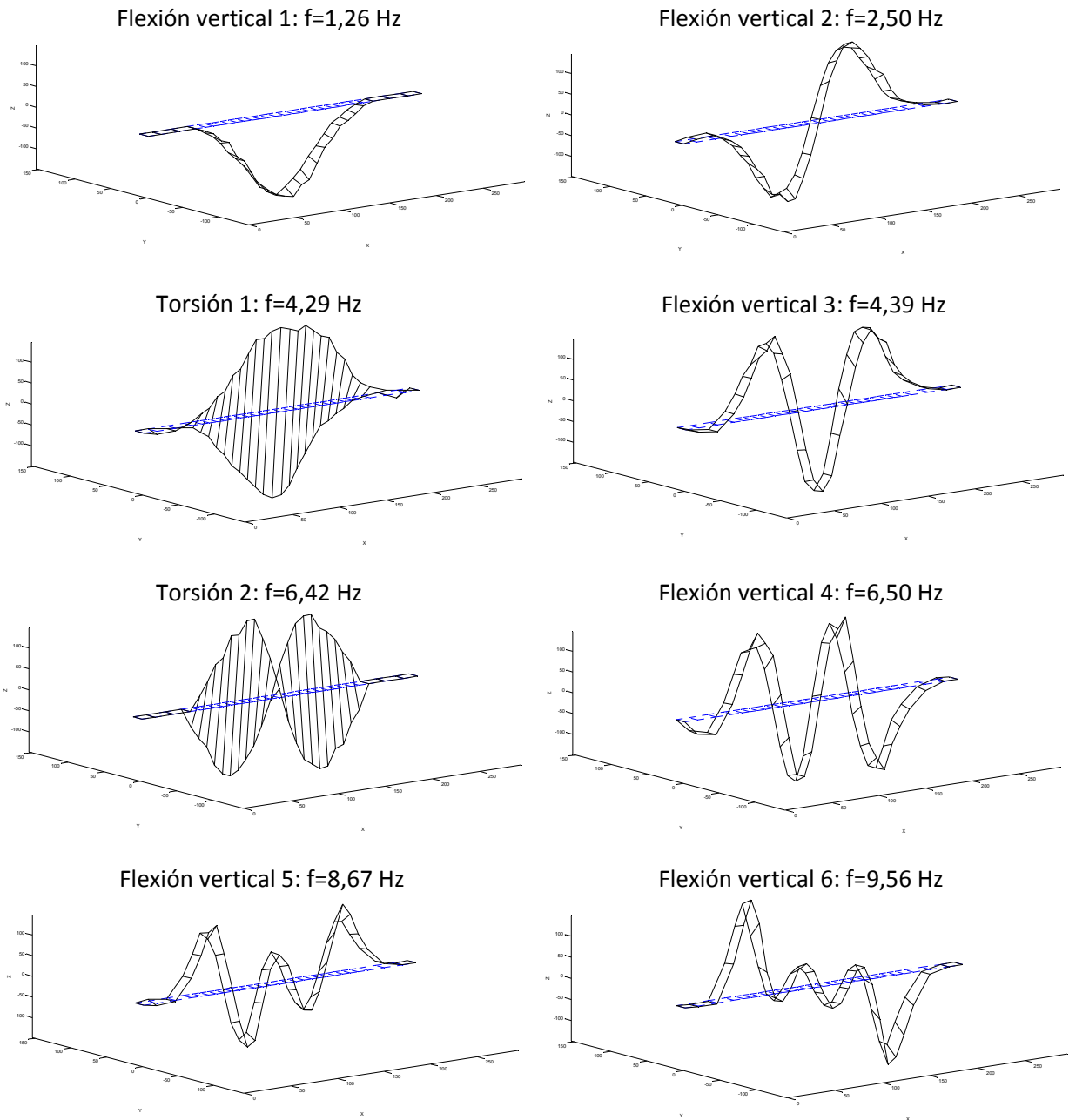
Figura 17. Ejemplo de formas modales experimentales identificadas (Garita-Durán, et. al., 2016).
