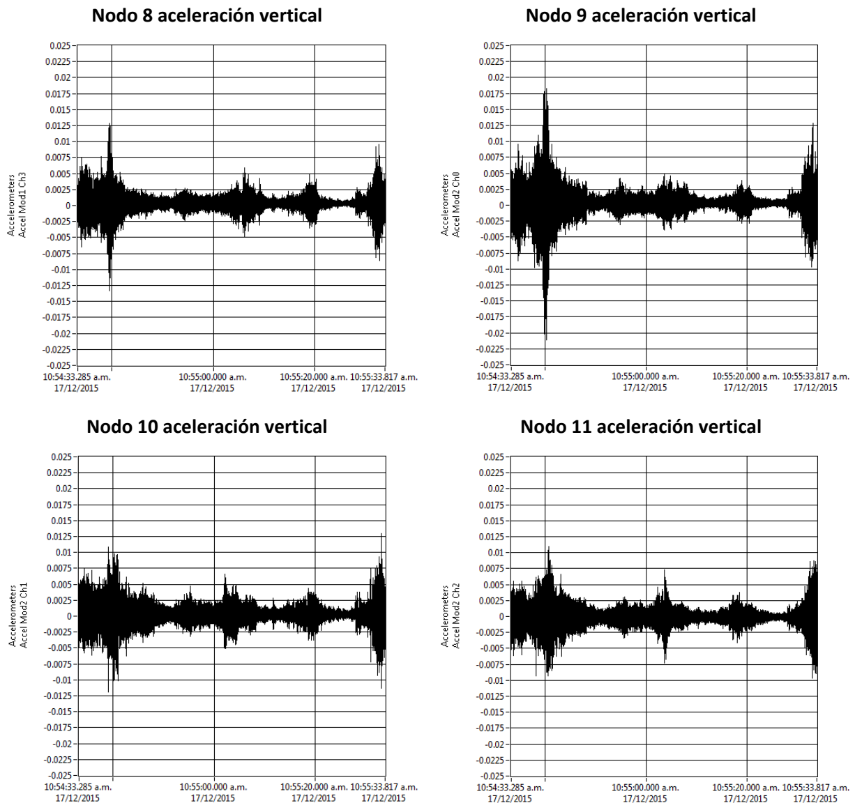
Figura 15. Registros de aceleración vertical del costado norte (config. 1 bloque 3).
