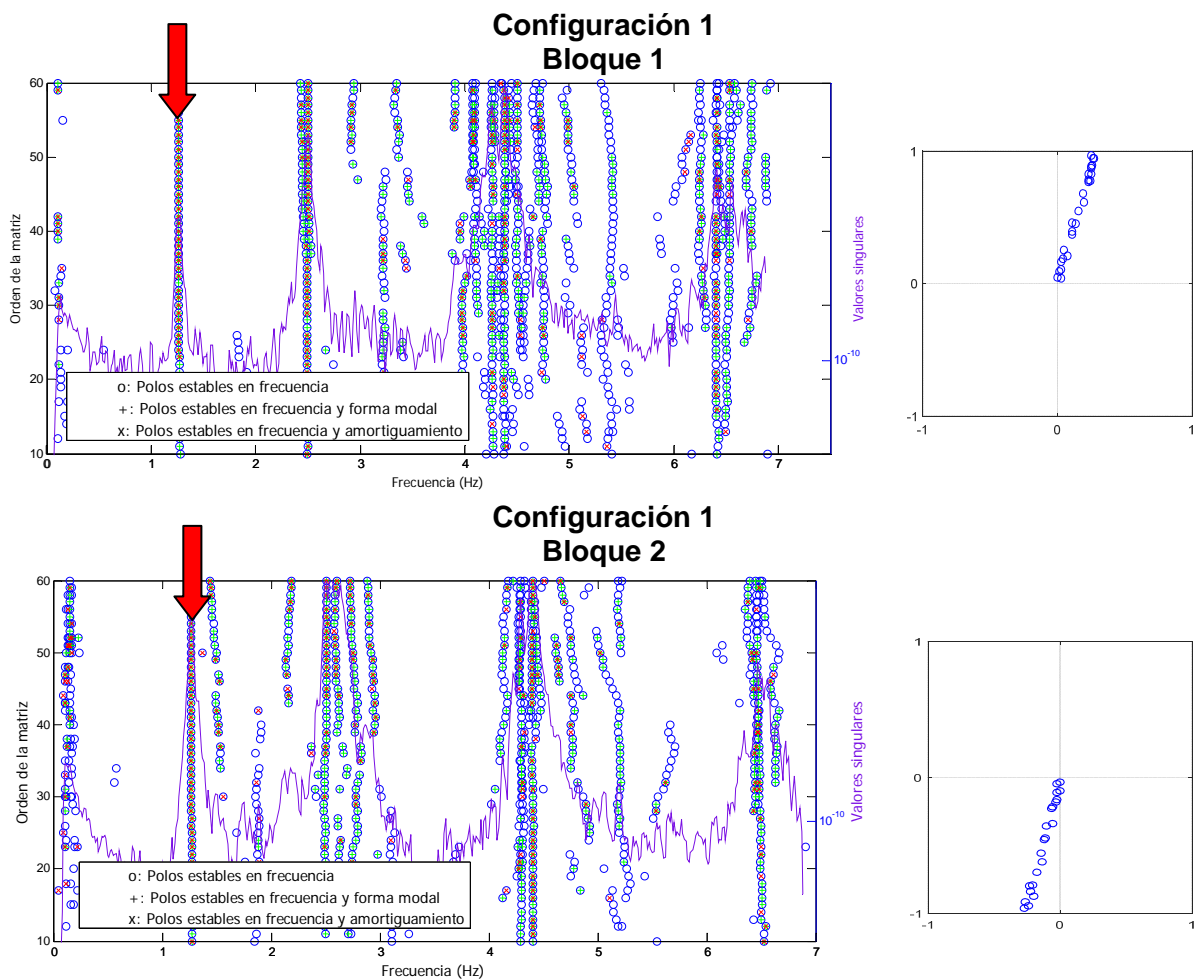
Figura 16. Diagrama de estabilización y diagrama de Argand correspondiente al modo 1, las flechas rojas indican el modo f=1,258 Hz (Garita-Durán, et. al., 2016).
