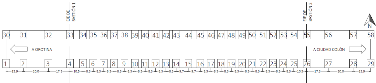
Figura 11. Numeración de nodos (Garita-Durán, et. al., 2016)
