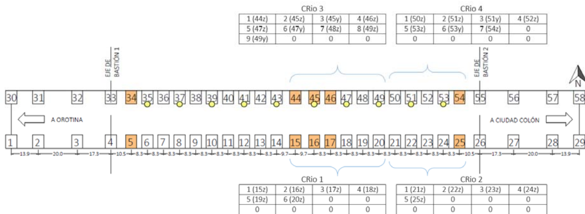
Figura 12. Distribución de sensores sobre el puente en la configuración 2 (Garita-Durán, et. al., 2016)
